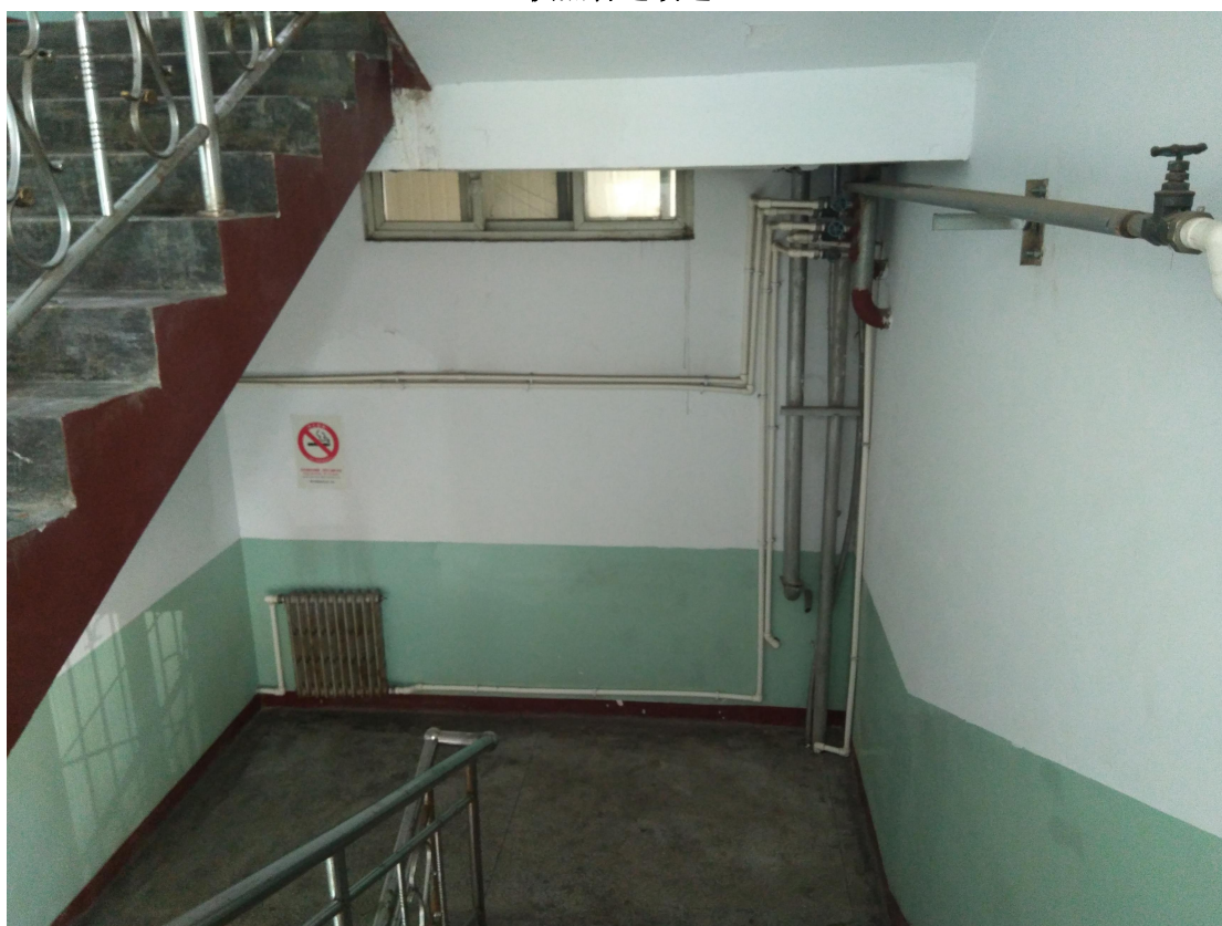
(供热管道改造)
